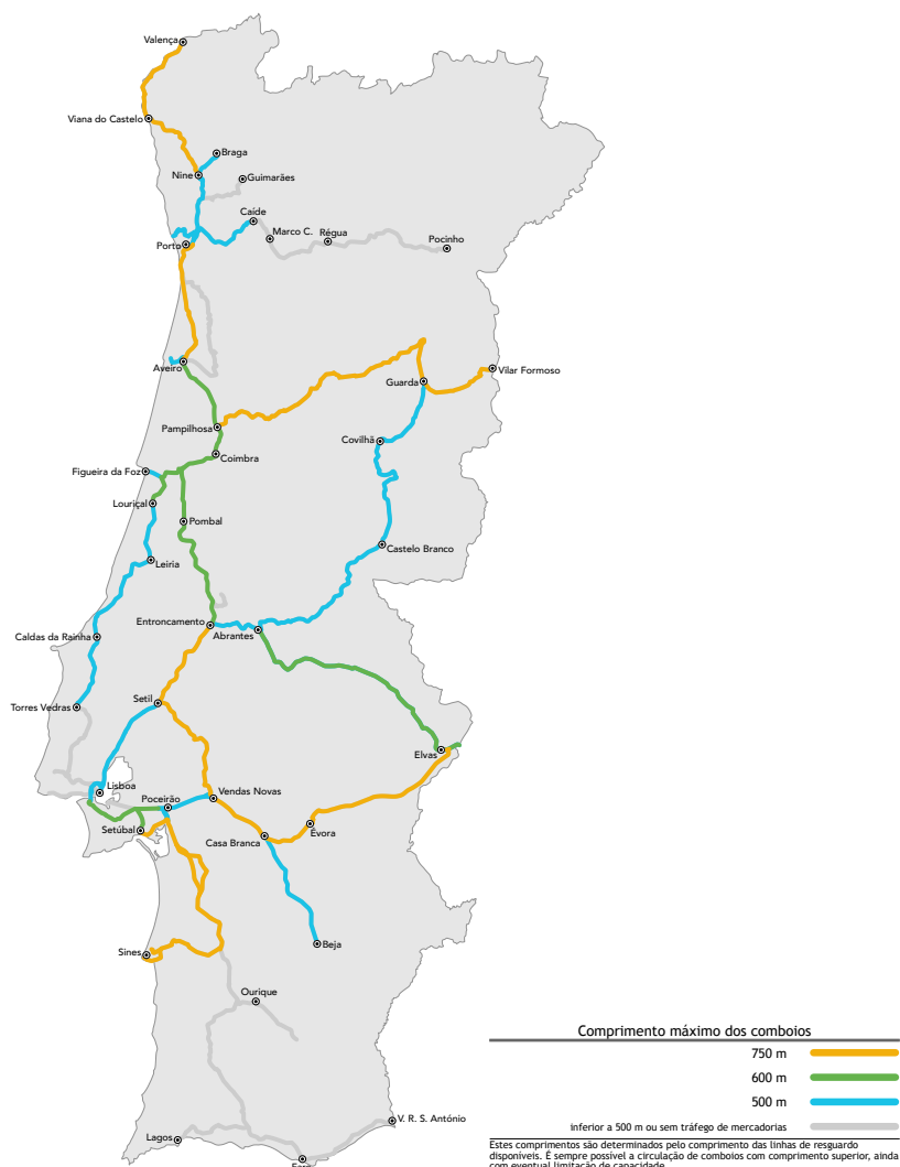
Figura 2. Comprimento máximo dos comboios de mercadorias na rede ferroviária após a conclusão do programa de investimentos Ferrovia 2020.
