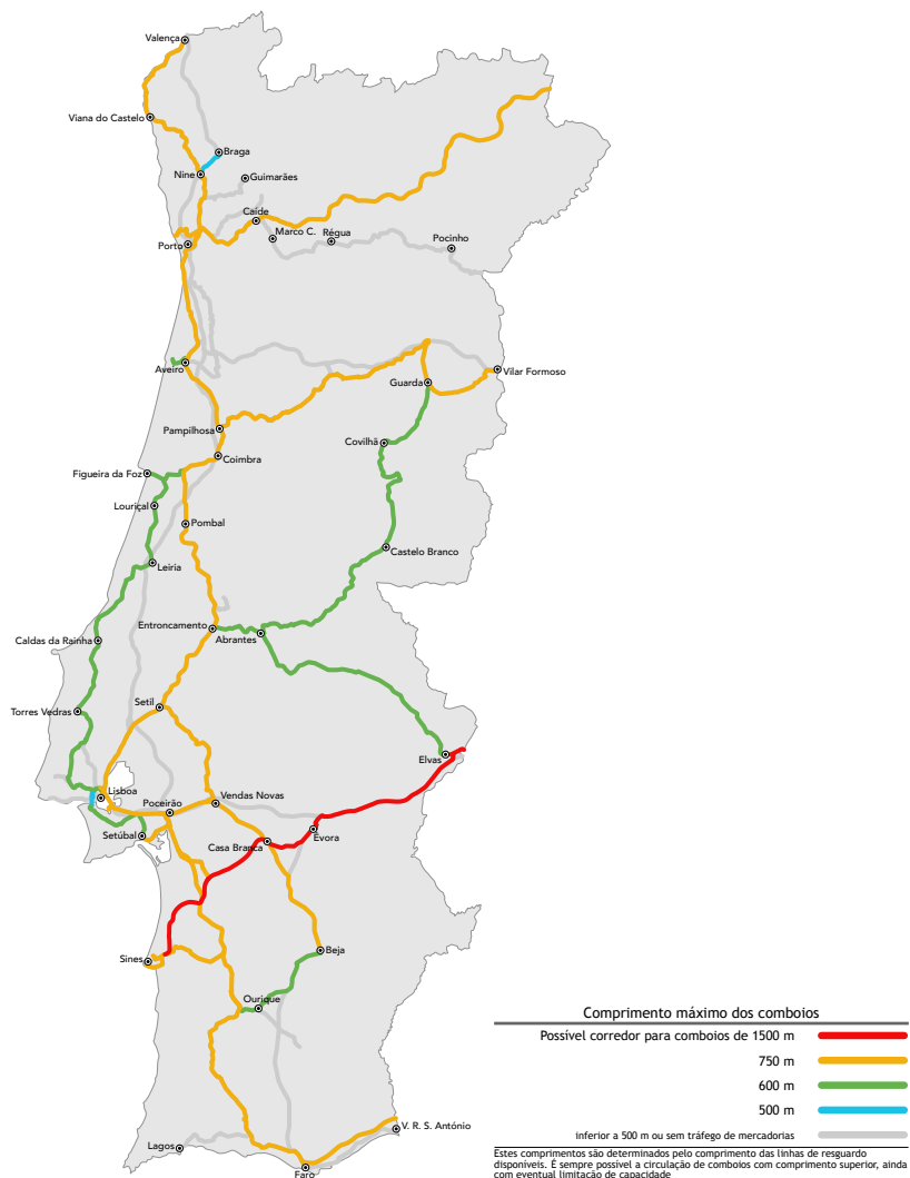
Figura 4. Comprimento máximo dos comboios de mercadorias na rede ferroviária com a criação de um possível corredor para comboios de 1500 m entre o Porto de Sines e a fronteira.
